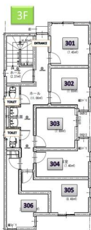
間取図
